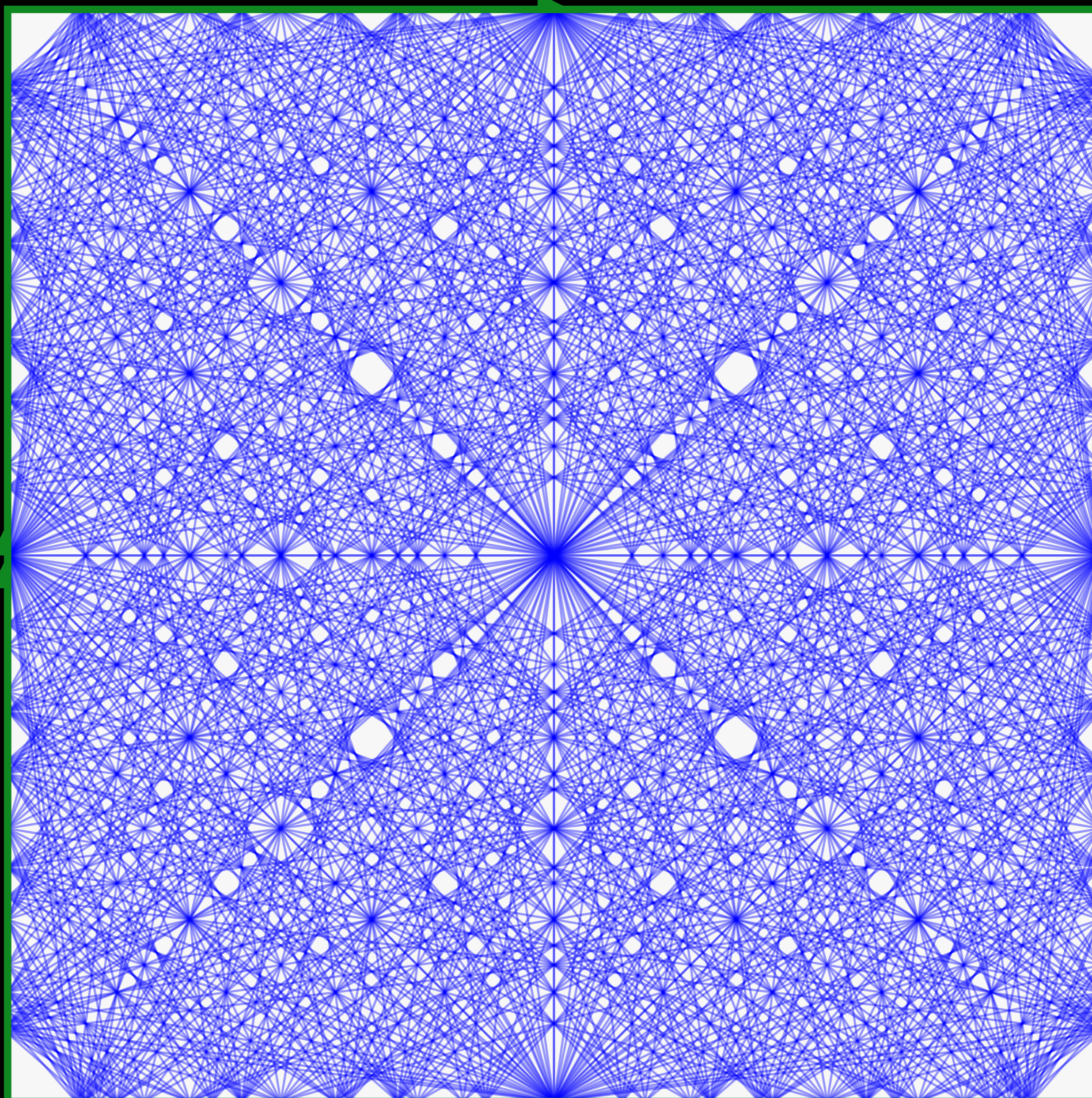
Euclidean torus
