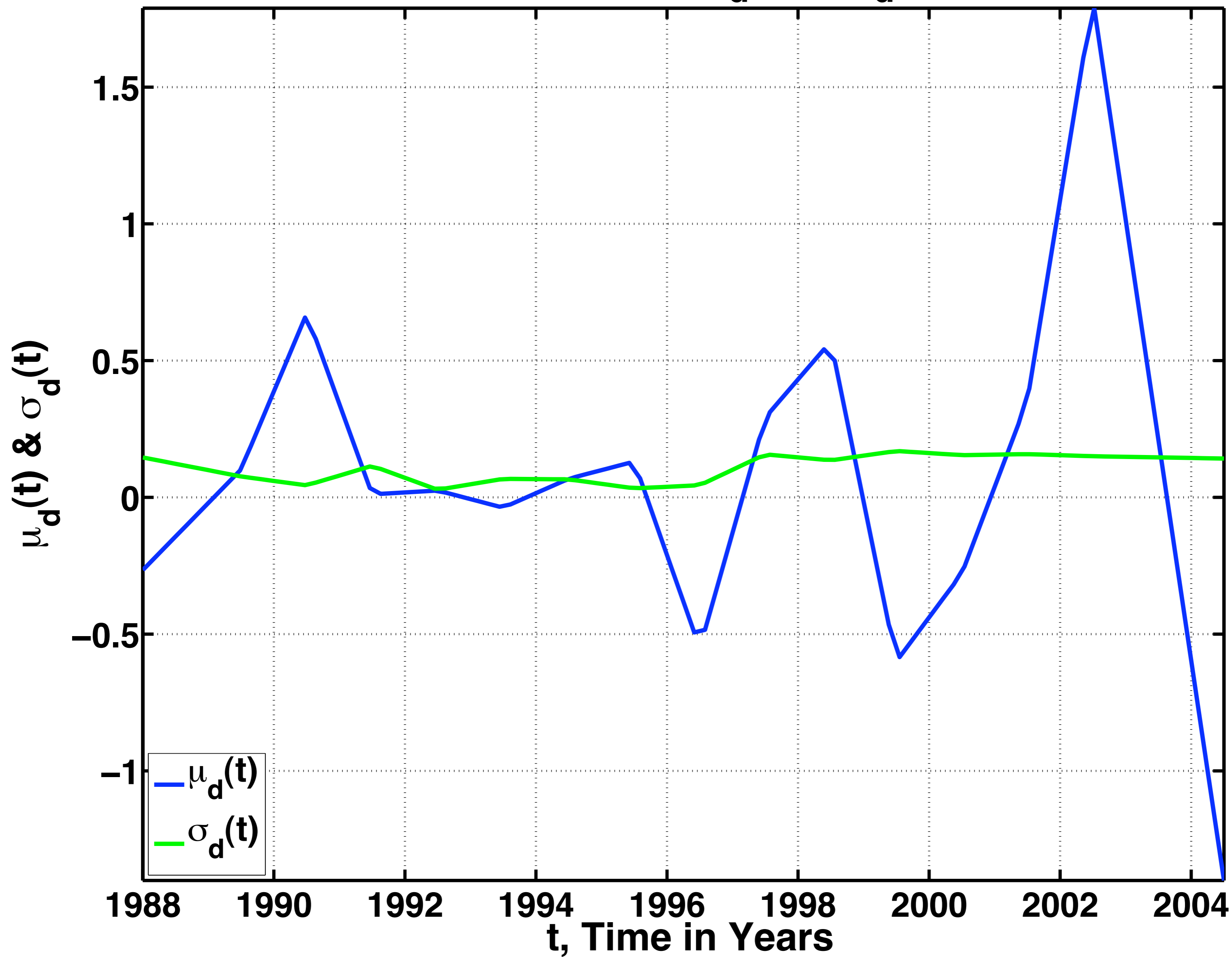
Diffusion Parameters: \mu_d(t) & \sigma_d(t) versus t
